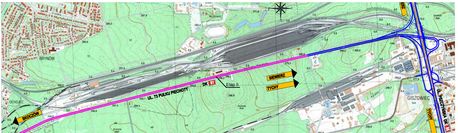
RYS. 3 DK 81: zadanie 4. Budowa węzła drogowego ul. 73. Pułku Piechoty, ul. Pszczyńskiej, ul. Kolistej i ul. Karolinki w Giszowcu – koszt 350 mln zł, udział Miasta – 175 mln zł (kolor niebieski); zadanie 5. Przebudowa ul. 73. Pułku Piechoty – koszt 100 mln zł, udział Miasta – 50 mln zł (kolor różowy).
