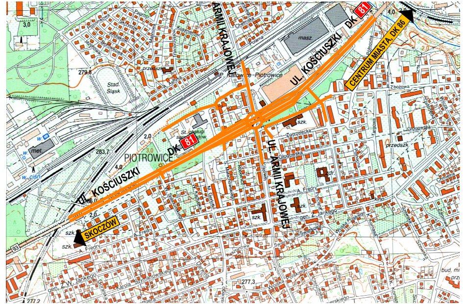
RYS. 2 DK 81: zadanie 3. Budowa dwupoziomowego skrzyżowania ul. Kościuszki i ul. Armii Krajowej – koszt 160 mln zł, udział Miasta – 80 mln zł (kolor pomarańczowy).
