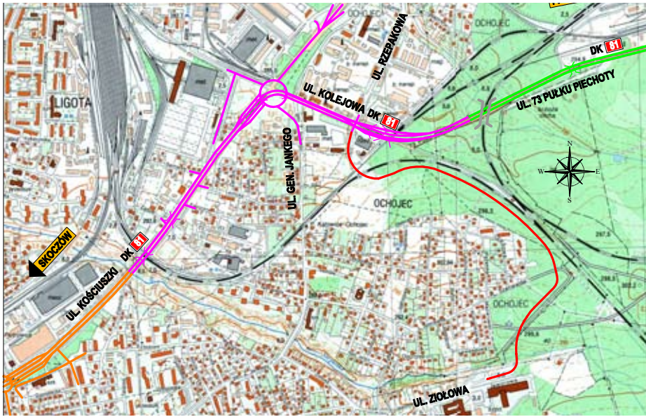
RYS. 1 DK 81: zadanie 1. Budowa węzła drogowego ul. Kościuszki, ul. Kolejowej, ul. Jankego oraz ul. Rzepakowej – koszt 630 mln zł, udział Miasta – 315 mln zł (kolor różowy); zadanie 2. Budowa połączenia ul. Kolejowej z ul. Ziołową – koszt 40 mln zł, udział Miasta – 20 mln zł (kolor czerwony).
